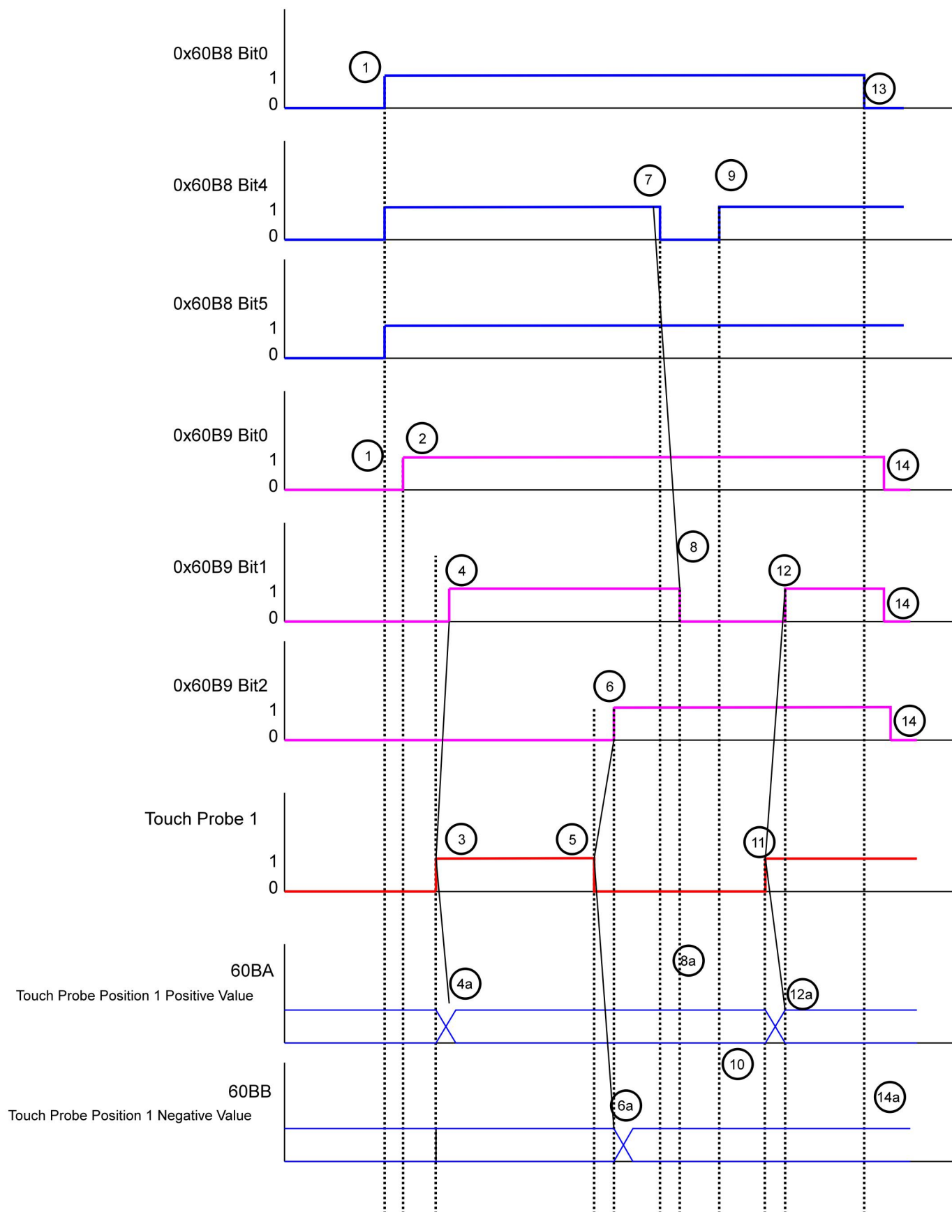
探针时序图
