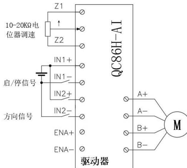
QC86H-AI 接线图
